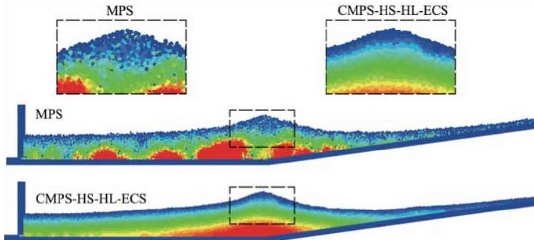
図-1 標準MPS法と高精度粒子法（CMPS-HS-HL-ECS法）による一様斜面上砕波のシミュレーション
