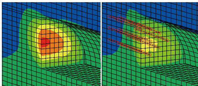
図-4 鏡ボルトによる変位抑制効果
