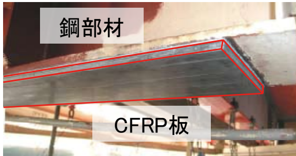
図-6 CFRP板接着工法
