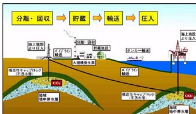
図-1 \text{CO}_2 地中貯留技術の概念図（RITE資料）
